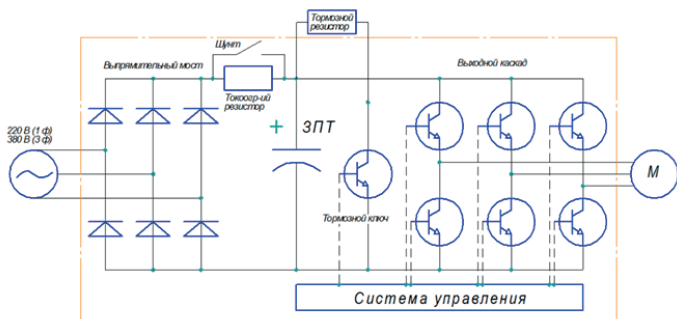
Рис. 2.1.1 Принципиальная электрическая схема ПЧ
